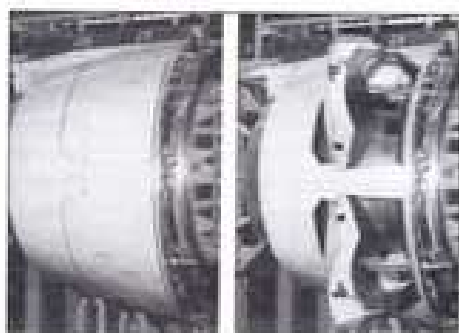
Inverseurs de poussée : à gauche portes fermées, à droite portes ouvertes
